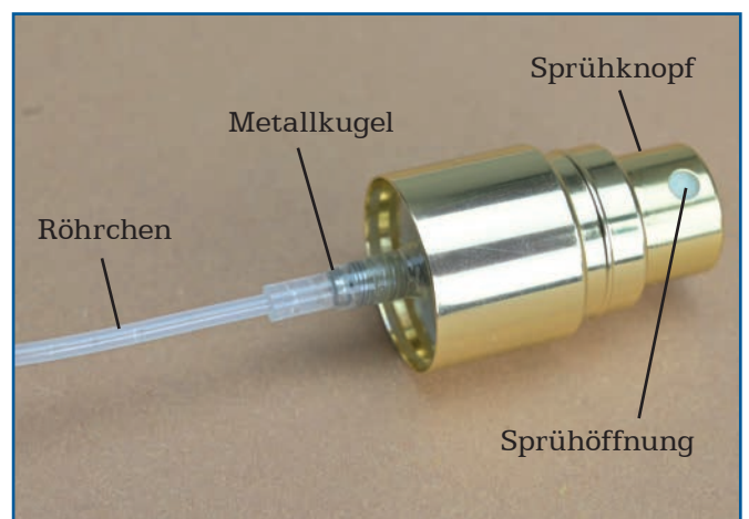
Abb. 2: abgeschraubter Sprühkopf
