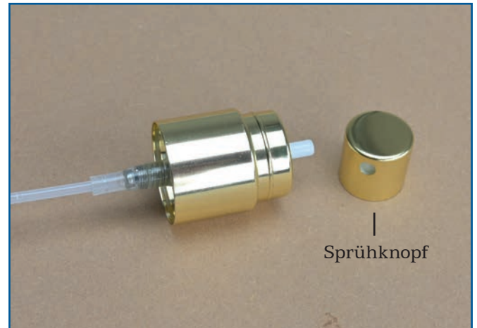
Abb. 3: abgezogener Sprühkopf
